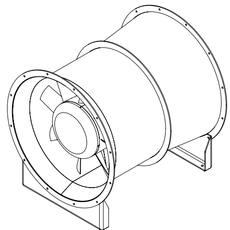
משקל מפוח ללא מנוע 150 ק"ג
