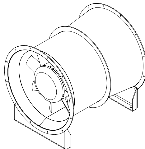
משקל מפוח ללא מנוע 115 ק"ג
