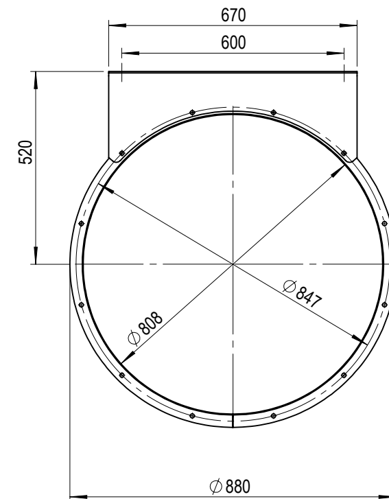
SECTION A-A
