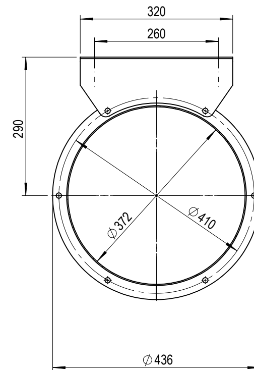
SECTION A-A
